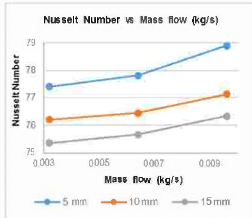
Gambar 6.8. Grafik hubungan Nusselt number dengan mass flow
