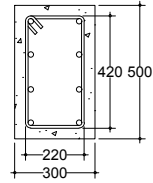
23 DIMENSI SLOOF DAN BALOK SCALE 1 : 10
