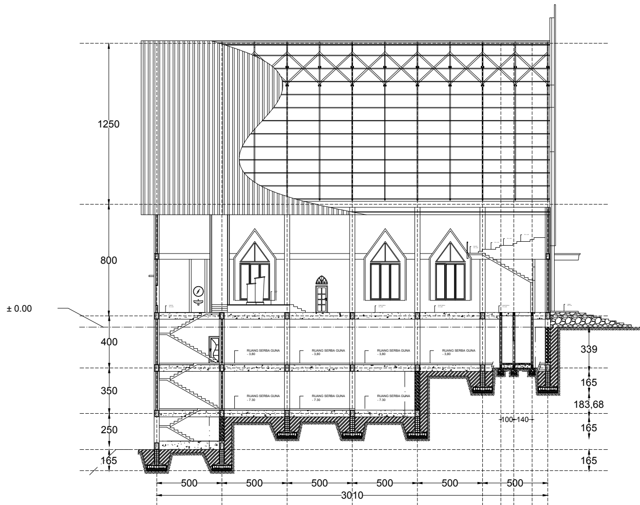
15 POTONGAN B-B SCALE 1 : 200
