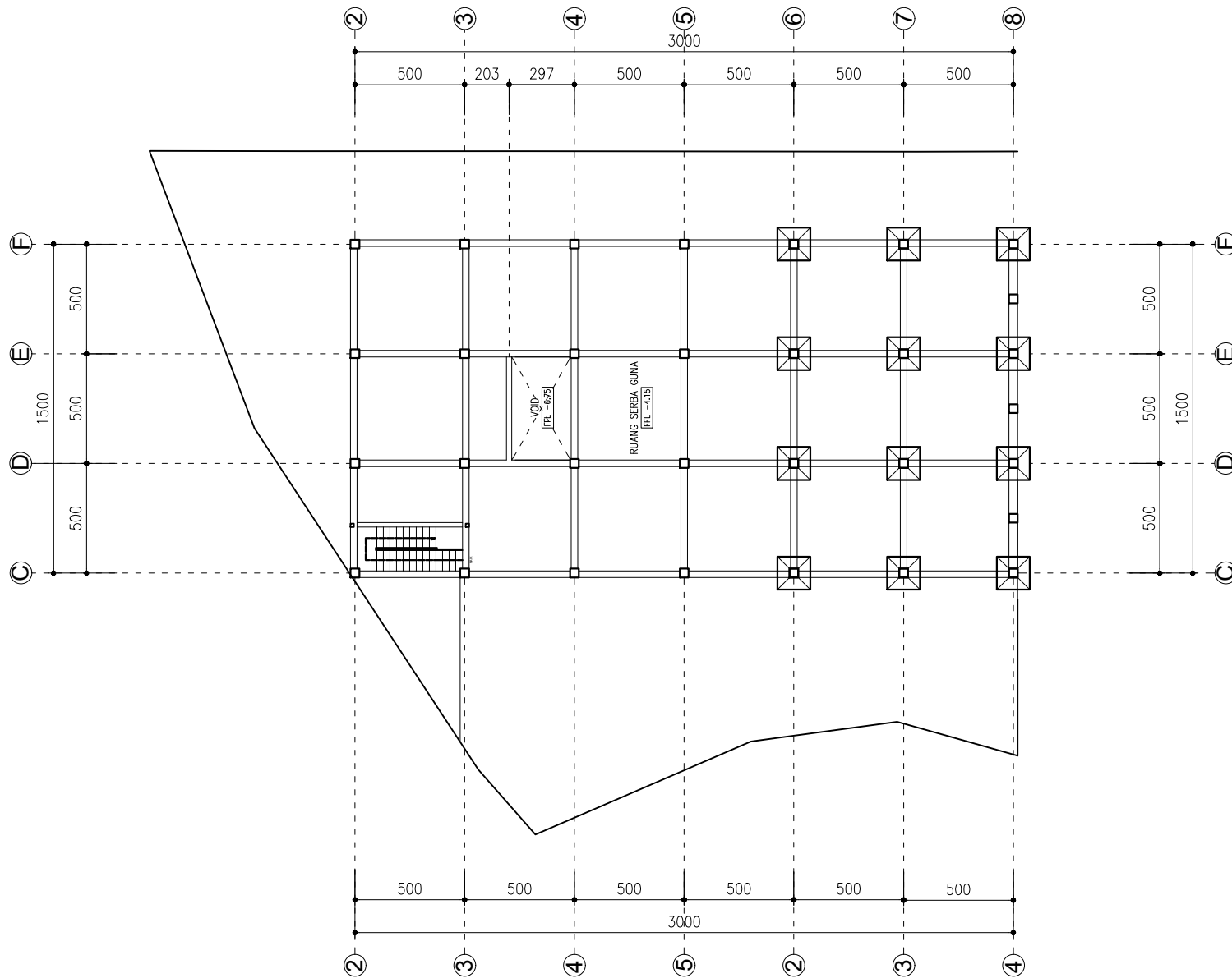
08 DENAH RENCANA PONDASI POER PLAT, SLOEF DAN RING BALK FFL 4.15(EL -78,15) SCALE 1 : 100
