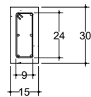
25 DIMENSI BALOK ANAK SCALE 1 : 10
