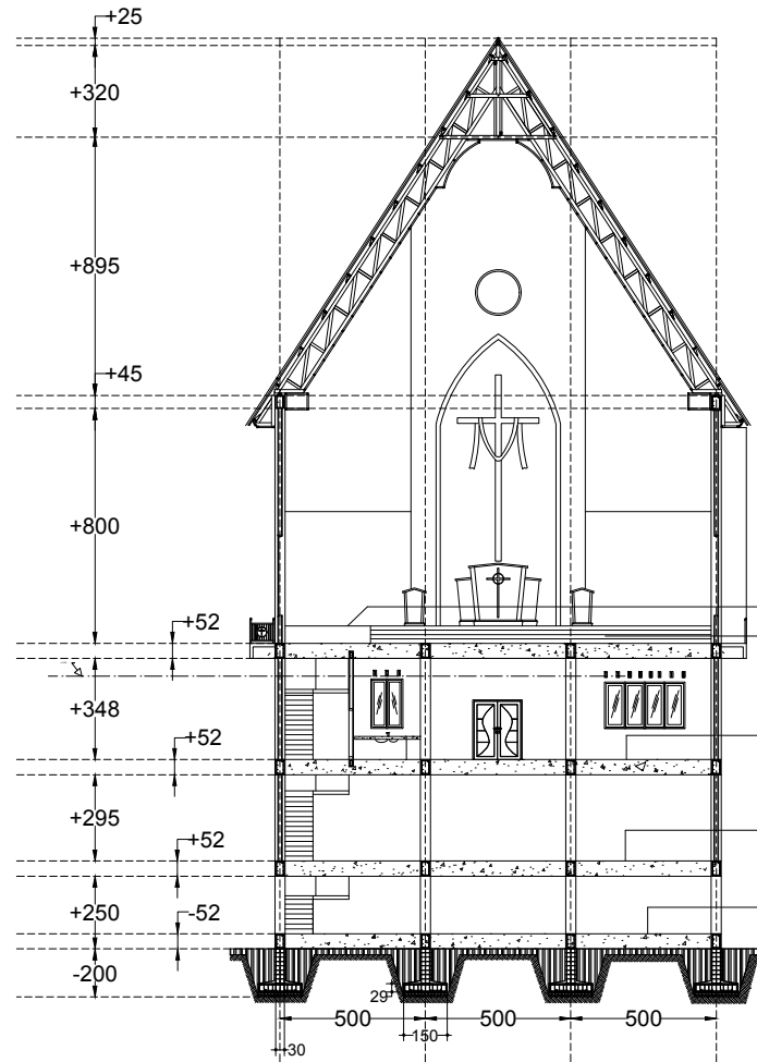
14 POTONGAN A-A SCALE 1 : 200
