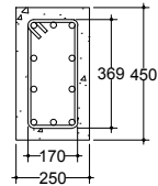
24 DIMENSI BALOK ANAK SCALE 1 : 10
