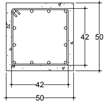
20 DIMENSI KOLOM UTAMA SCALE 1 : 10
