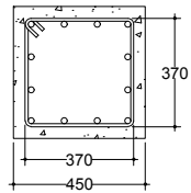
21 DIMENSI KOLOM ANAK SCALE 1 : 10
