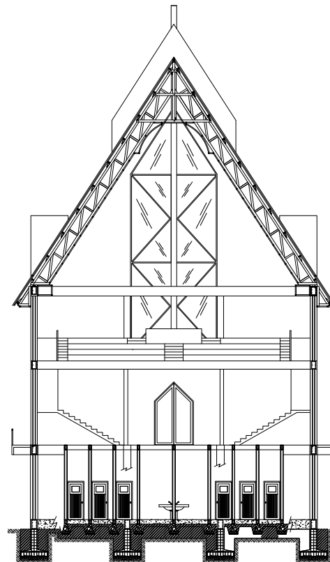
16 POTONGAN C-C - SCALE 1 : 200
