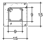
22 DIMENSI KOLOM PRAKTIS SCALE 1 : 10
