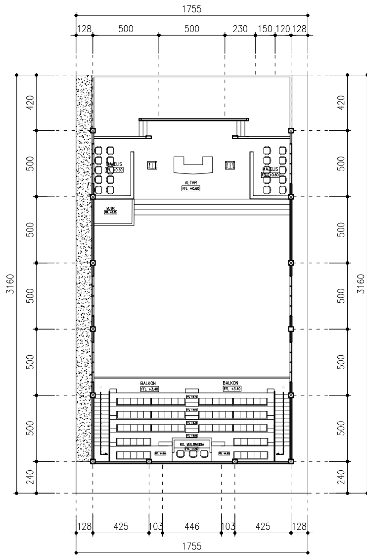
05 DENAH BALKON SCALE 1 : 100
