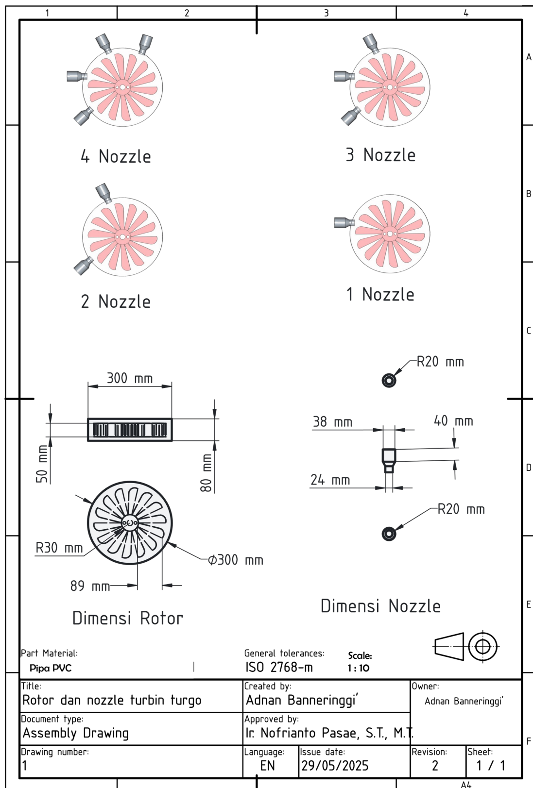
Gambar L.3 Rotor Dan Nozzle Turbin Turgo
