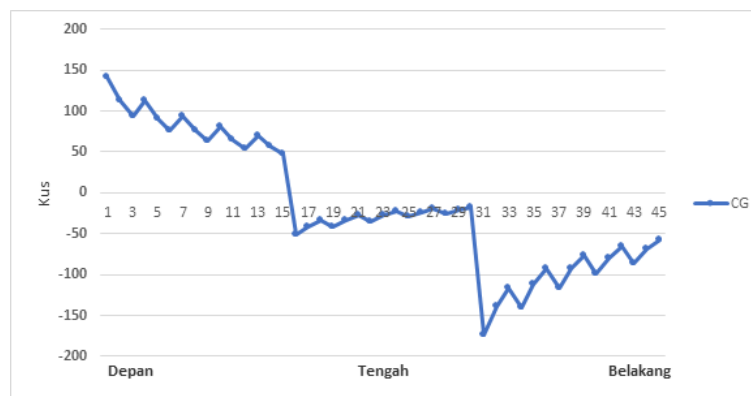
Gambar 4. Grafik index understeer (Kus)
