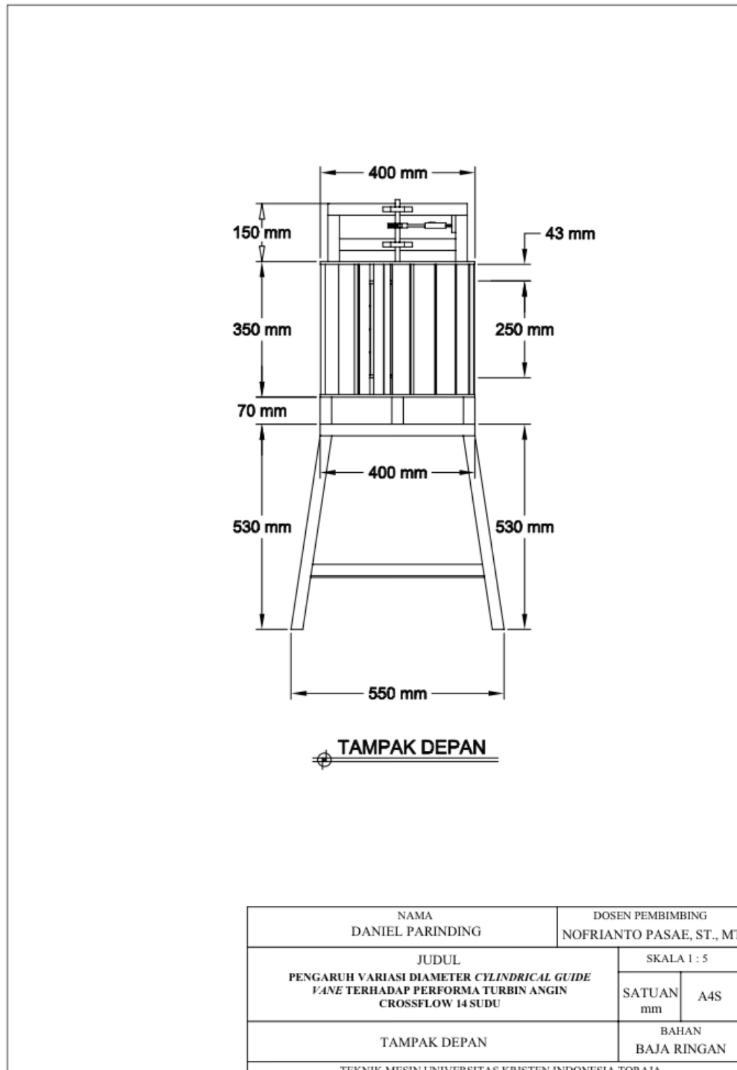
Gambar L. 8 Tampak depan Cylindrical guide vane 400 mm
