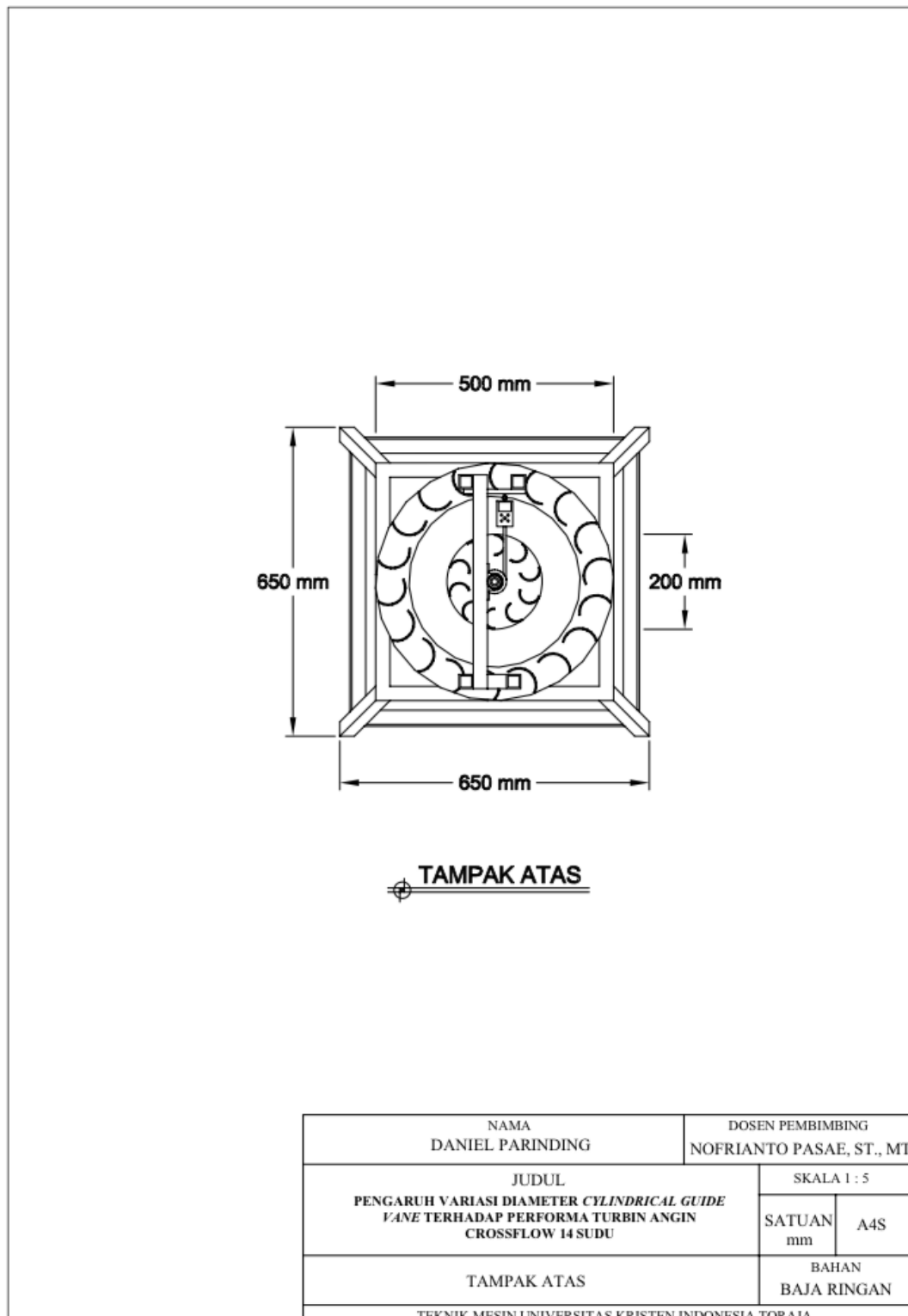
Gambar L. 12 Tampak atas Cylindrical guide vane 500 mm
