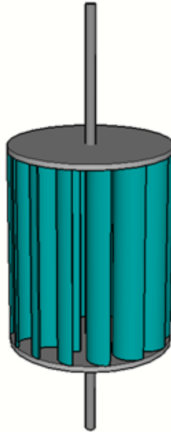
Gambar L. 5 Rotor Turbin Angin Crossflow 14 sudu
