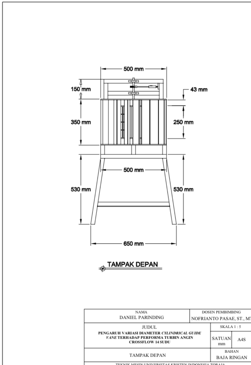
Gambar L. 6 Tampak depan Cylindrical guide vane 500 mm
