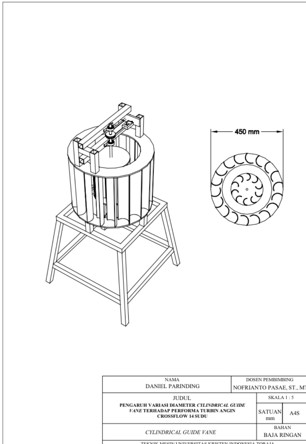
Gambar L. 10 Cylindrical guide vane 450 mm
