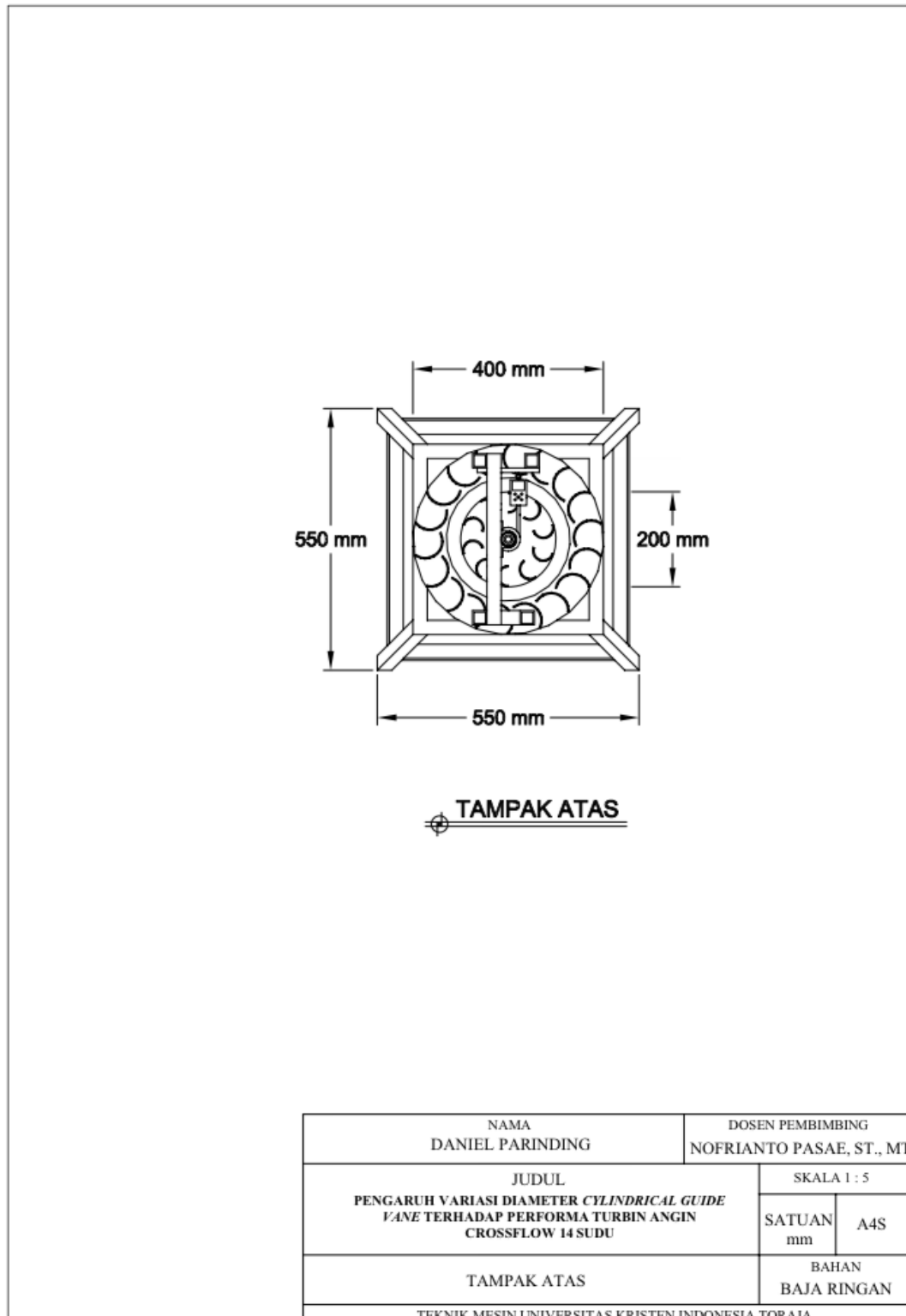
Gambar L. 14 Tampak atas Cylindrical guide vane 400 mm
