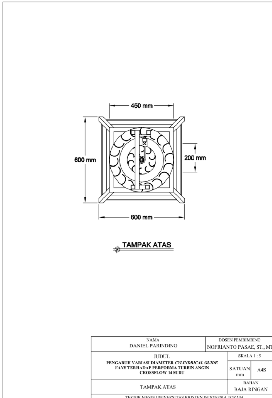
Gambar L. 13 Tampak atas Cylindrical guide vane 450 mm
