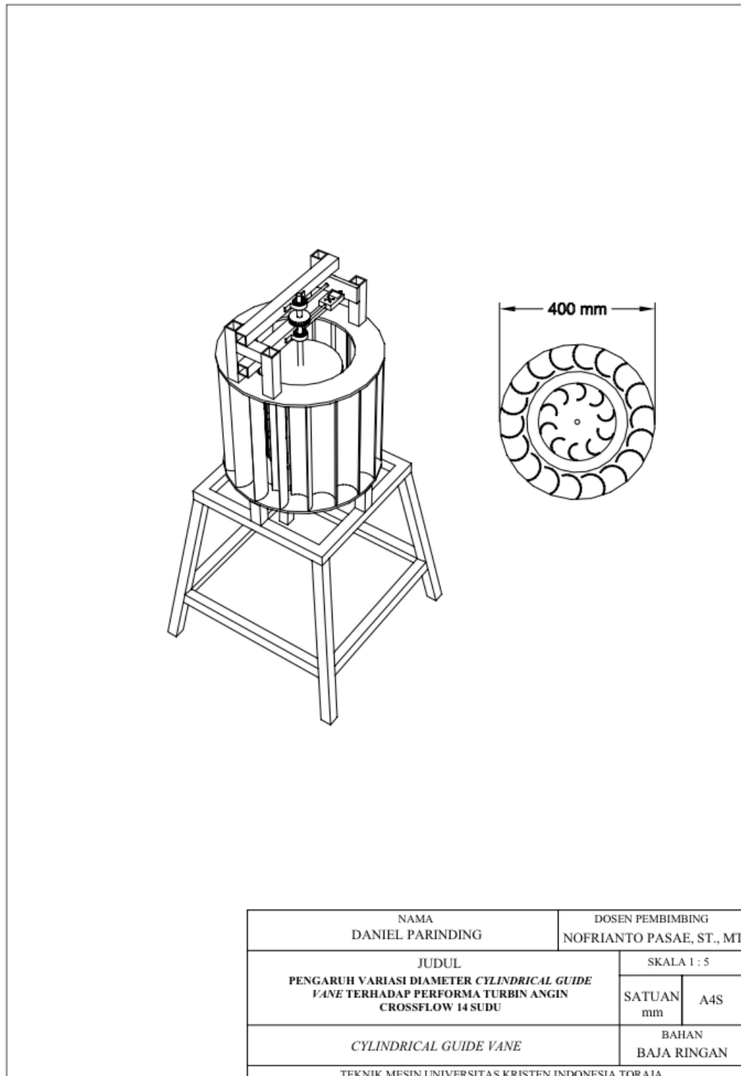
Gambar L. 11 Cylindrical guide vane 400 mm
