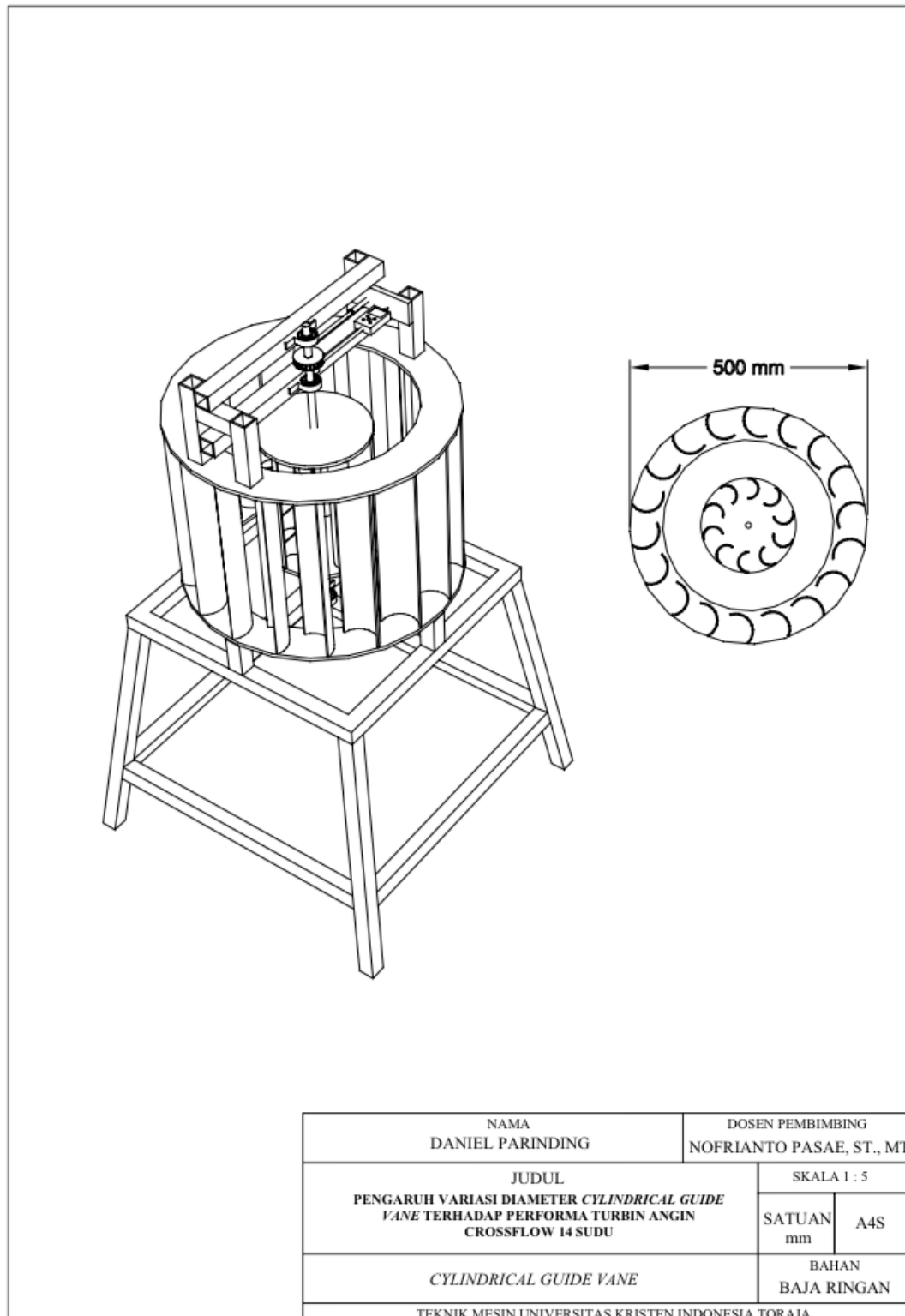
Gambar L. 9 Cylindrical guide vane 500 mm
