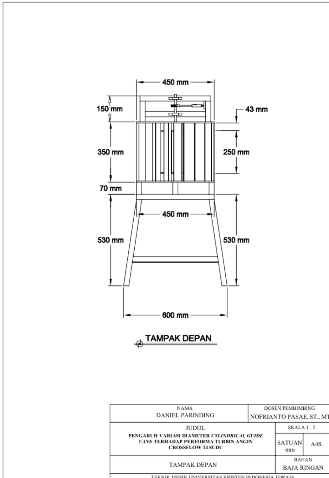
Gambar L. 7 Tampak depan Cylindrical guide vane 450 mm
