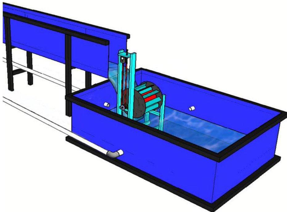
Gambar L.3 Layout kincir air pitchback dengan variasi sudut sudu model melengkung
