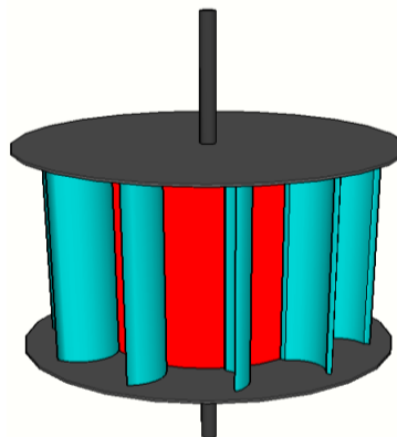
Gambar L.7 Rotor kincir air pitchback 10 sudu model melengkung dengan kemiringan sudu , 180^\circ
