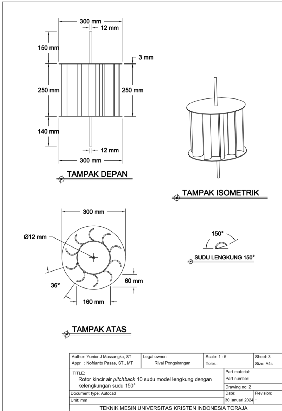
Gambar L.9 Rotor kincir air pitchback 10 sudu model melengkung dengan kemiringan sudu 150°
