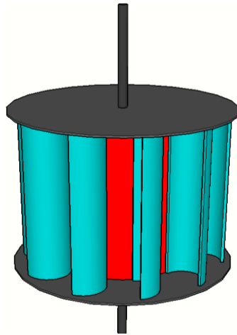
Gambar L.5 Rotor kincir air pitchback 10 sudu model melengkung dengan kemiringan sudu 120^\circ
