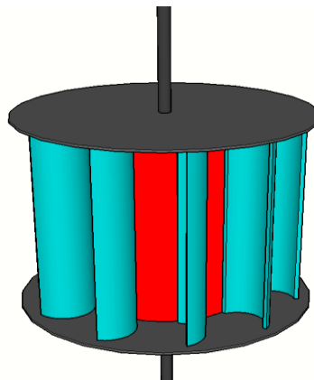
Gambar L.6 Rotor kincir air pitchback 10 sudu model melengkung dengan kemiringan sudu 150^\circ
