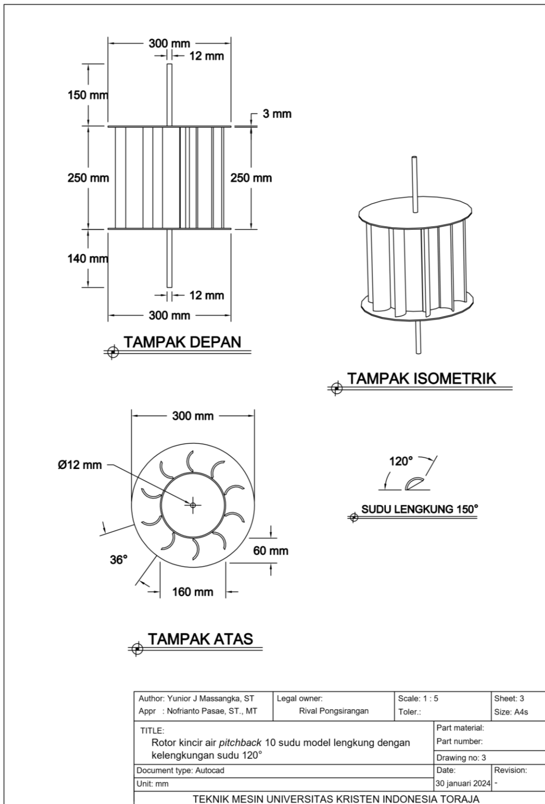
Gambar L.8 Rotor kincir air pitchback 10 sudu model melengkung dengan kemiringan sudu 120°
