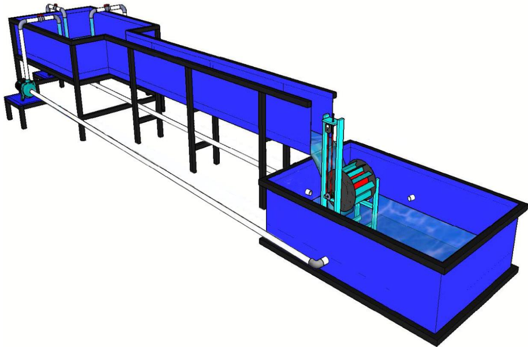
Gambar L.3 Layout kincir air pitchback dengan variasi sudut sudu model melengkung
