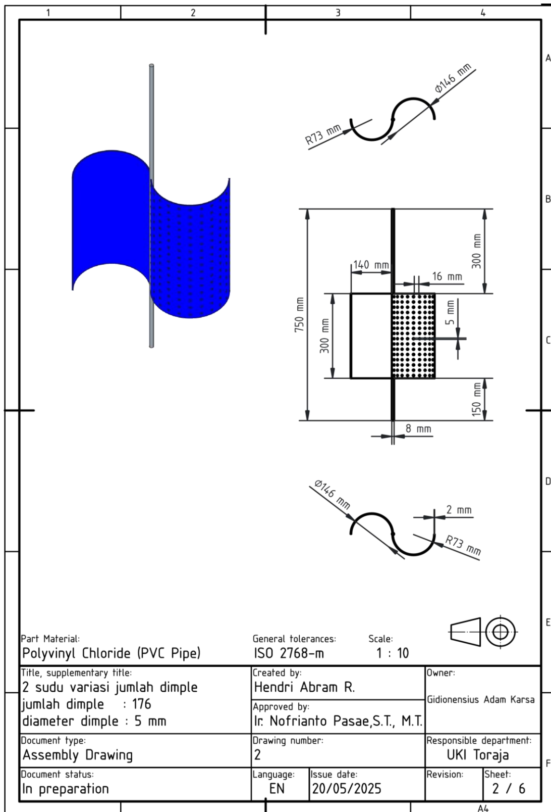
Gambar L.4 Dua Sudu Jumlah Dimple 352
