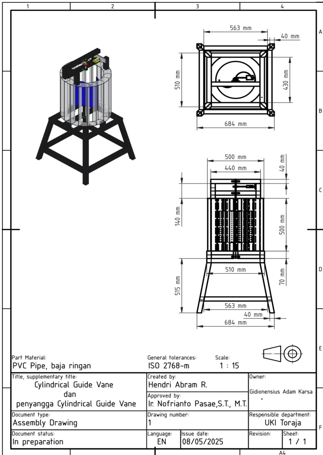
Gambar L.2 Rangka Cylindrical Guide Vane
