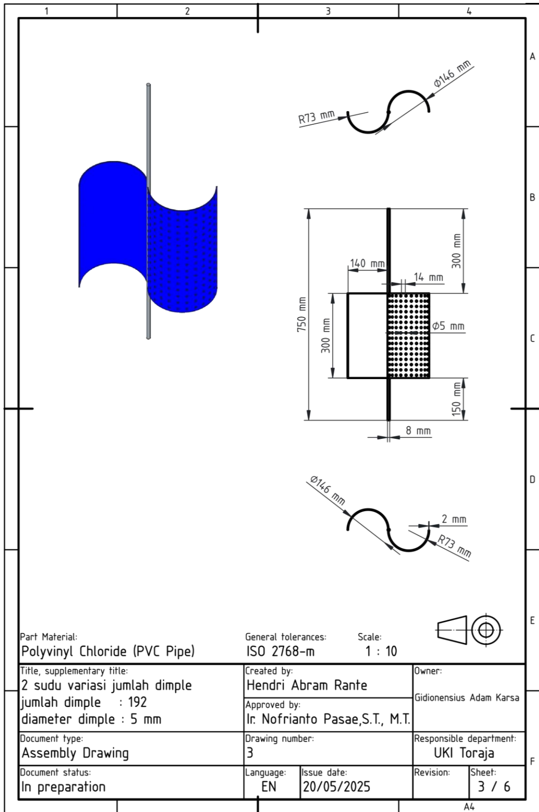
Gambar L.5 Dua Sudu Jumlah Dimple 384
