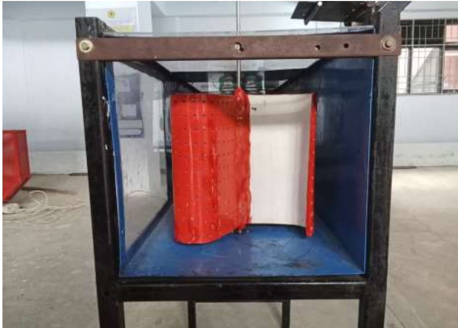
Gambar L.4 Turbin angin Savonius tiga sudu tampak belakang
