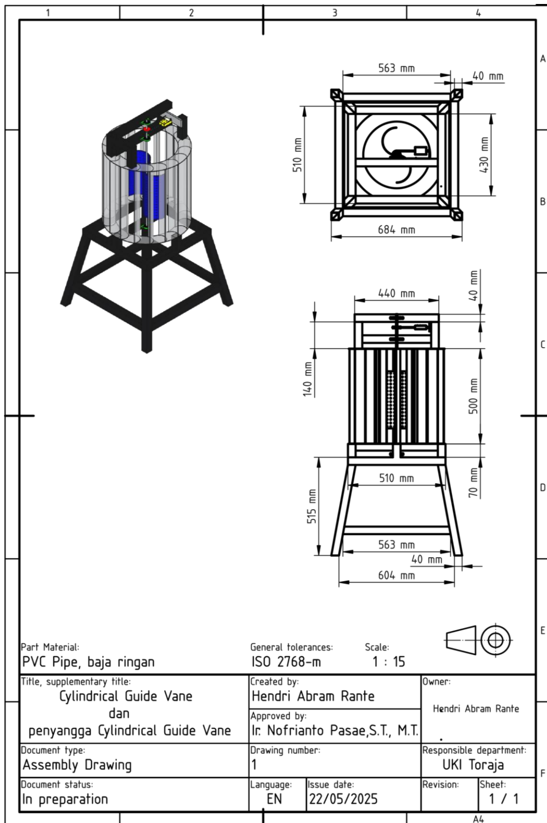
Gambar L.2 Rangka cylindrical guide vane
