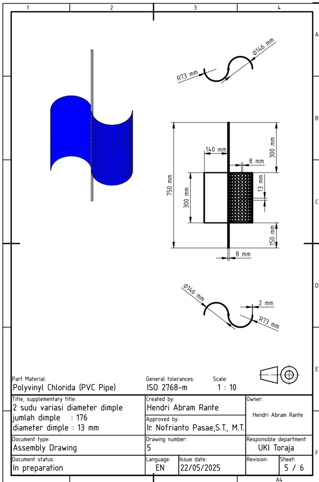
Gambar L.7 Dua sudu diameter dimple 13 mm
