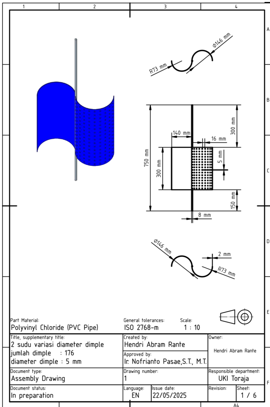
Gambar L.3 Dua sudu diameter dimple 5 mm
