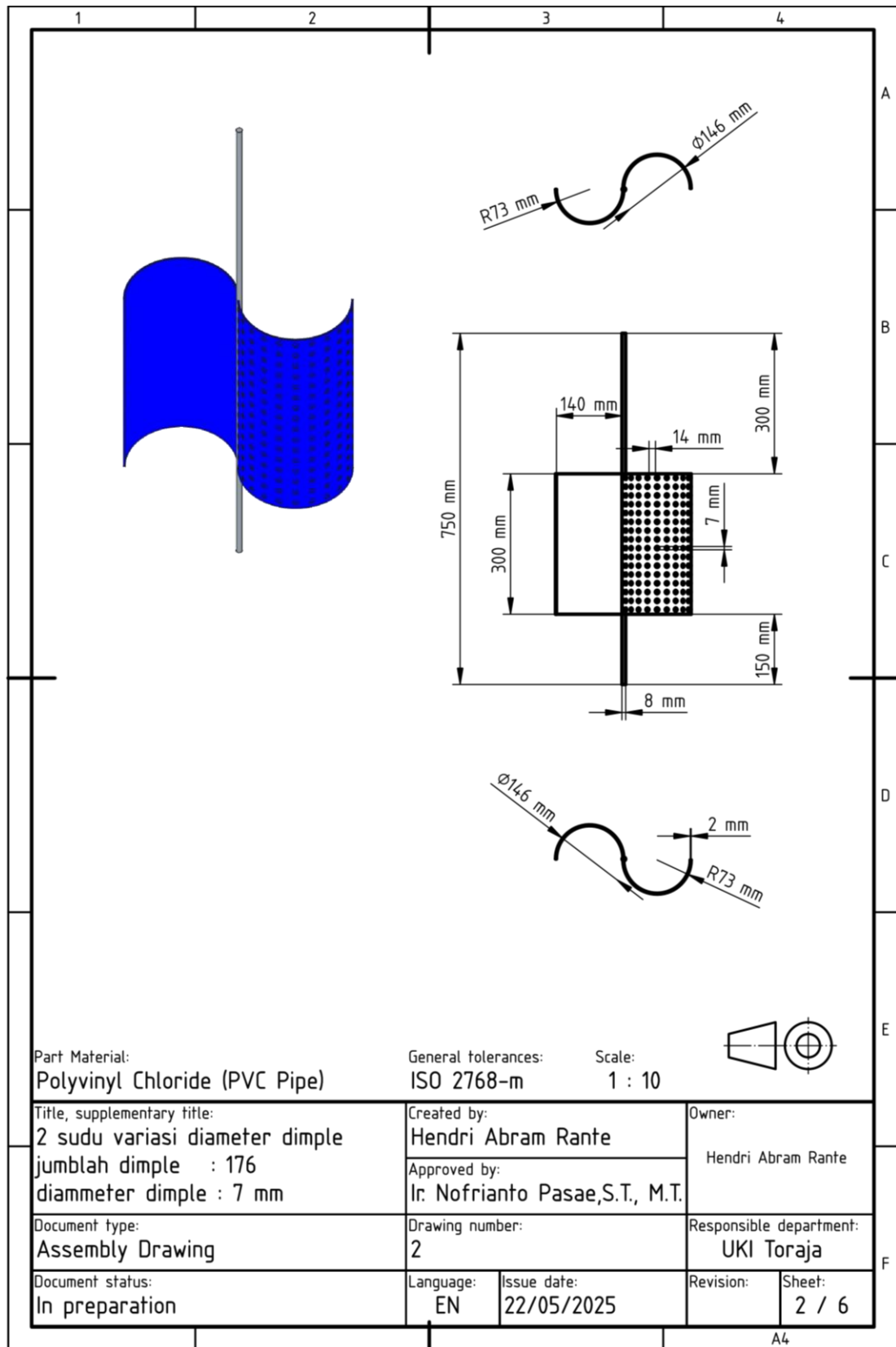
Gambar L.4 Dua sudu diameter dimple 7 mm
