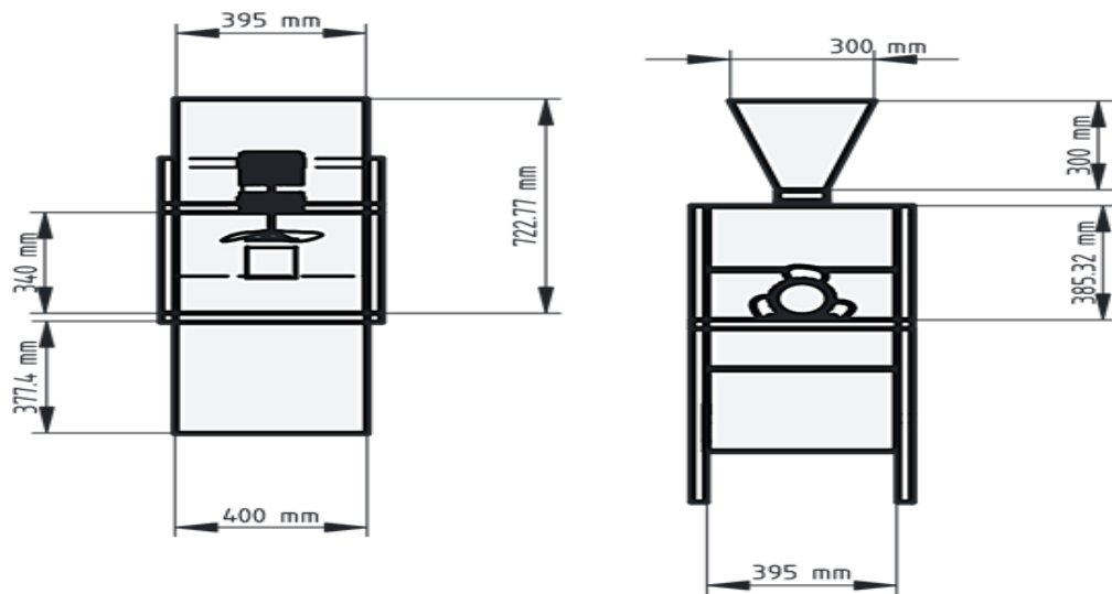
Gambar L-3 Desain 2 dimensi pembersih gabah tampak atas dan depan
