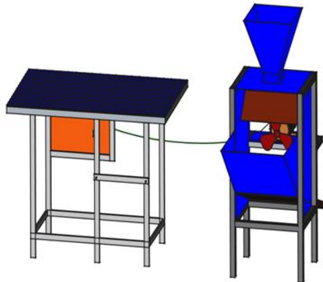
Gambar L-2 Desain 3 dimensi tampak belakang pembersih gabah
