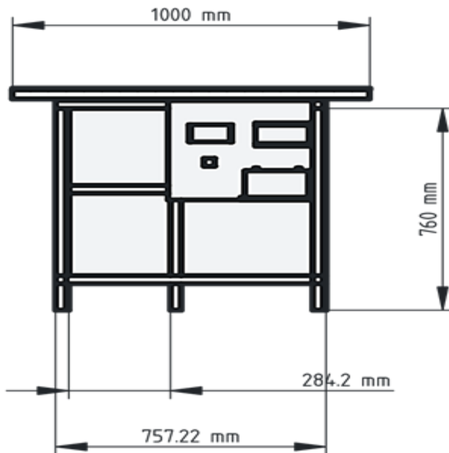
Gambar L-4 Ukuran Meja panel Surya 2 dimensi
