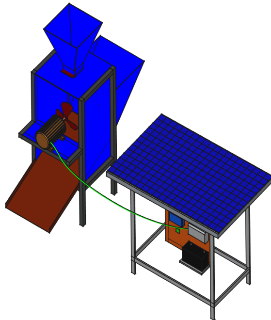
Gambar L-1 Desain 3 tampak depan pembersih gabah
