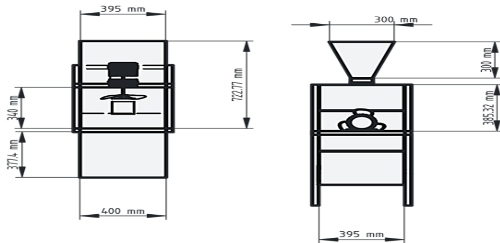
Gambar L-3 Desain 2 dimensi pembersih gabah tampak atas dan depan
