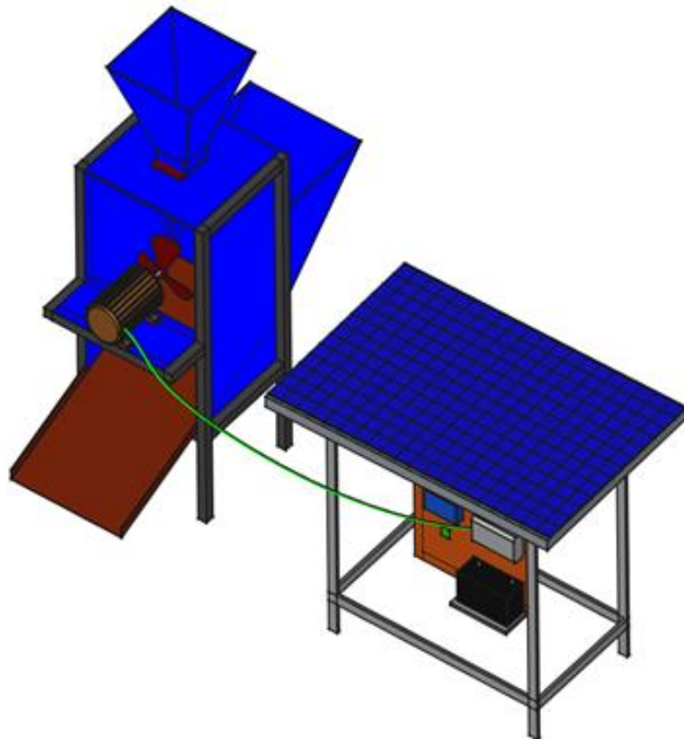
Gambar L-1 Desain 3 dimensi tampak depan pembersih gabah
