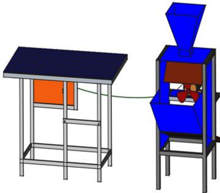
Gambar L-2 Desain 3 dimensi tampak belakang pembersih gabah
