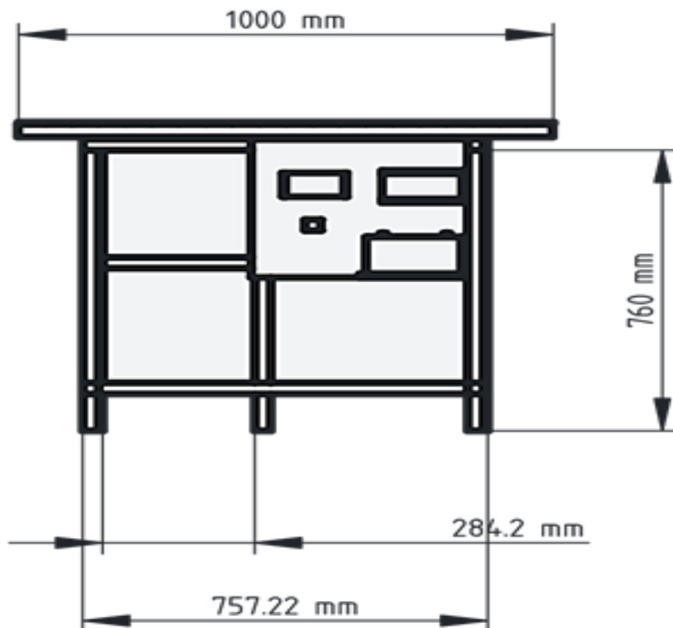
Gambar L-4 Ukuran meja panel surya 2 dimensi
