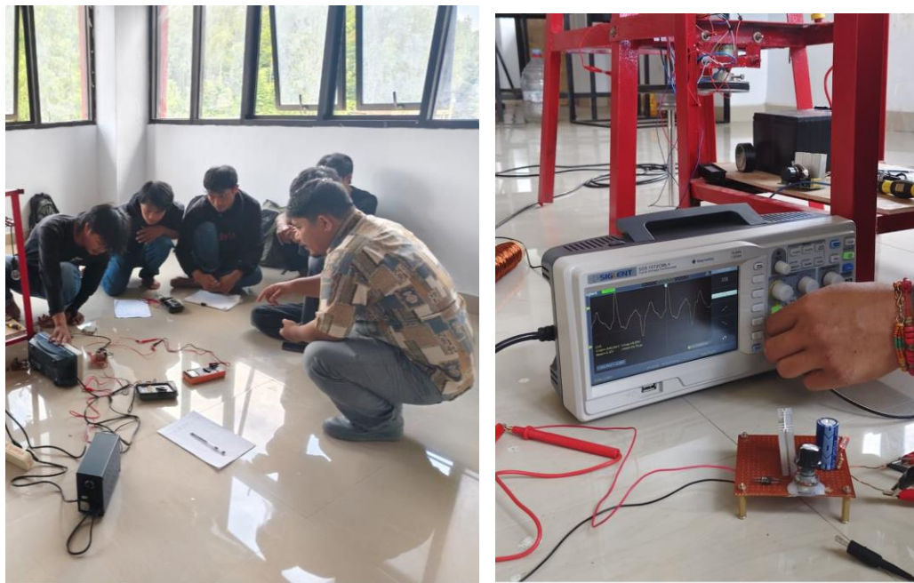
Gambar L-2.1 Pengukuran gelombang dengan menggunakan alat ukur osiloskop
